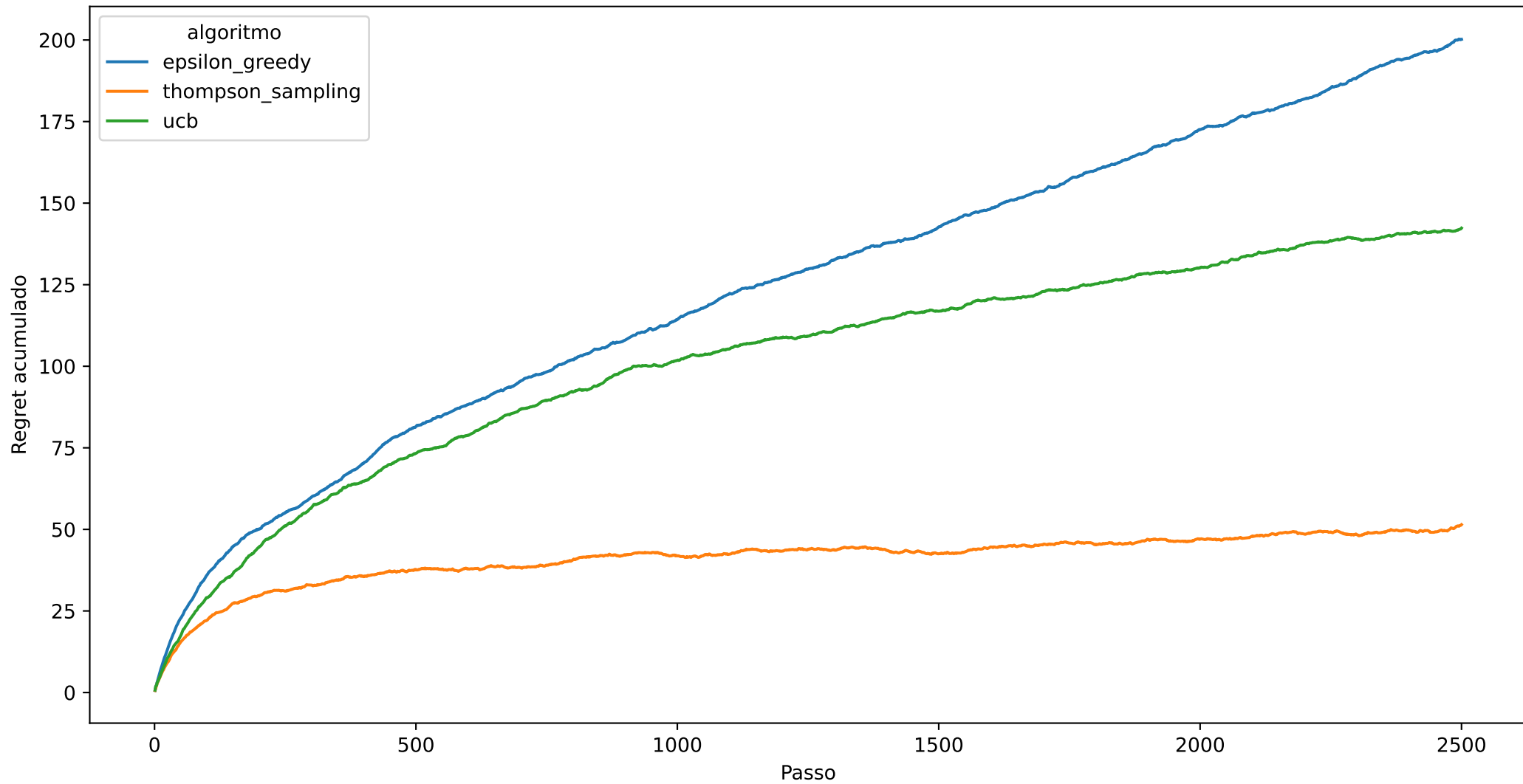
Bandit — Regret acumulado por algoritmo
